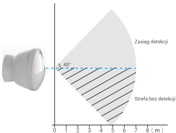
Rys. 2 Widok z góry zasięgu detekcji
