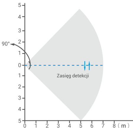
Rys. 2 Widok z góry zasięgu detekcji
