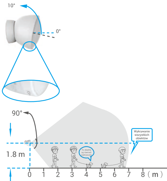
Rys. 1 Widok z boku zasięgu detekcji
